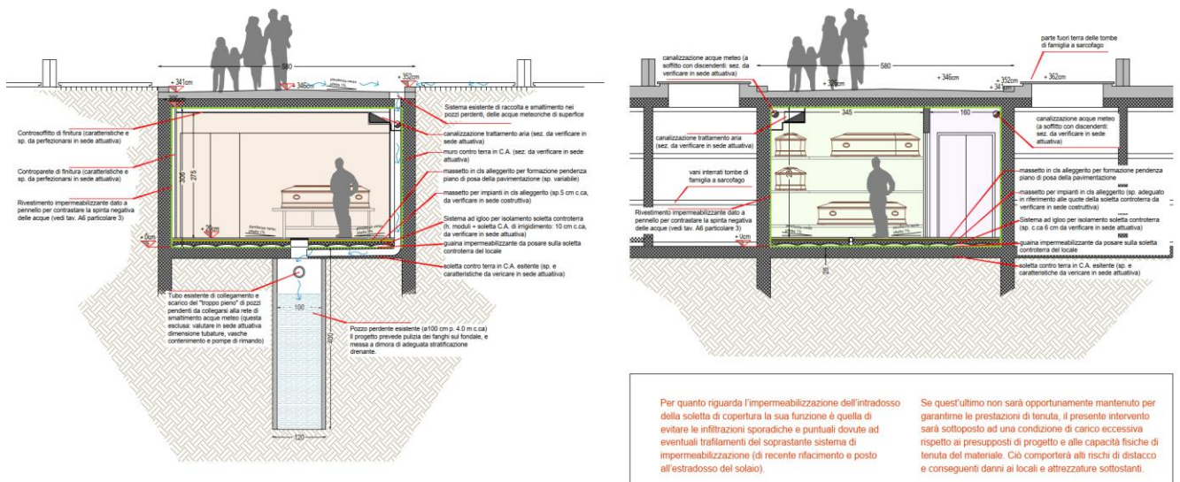
Sezioni di progetto
