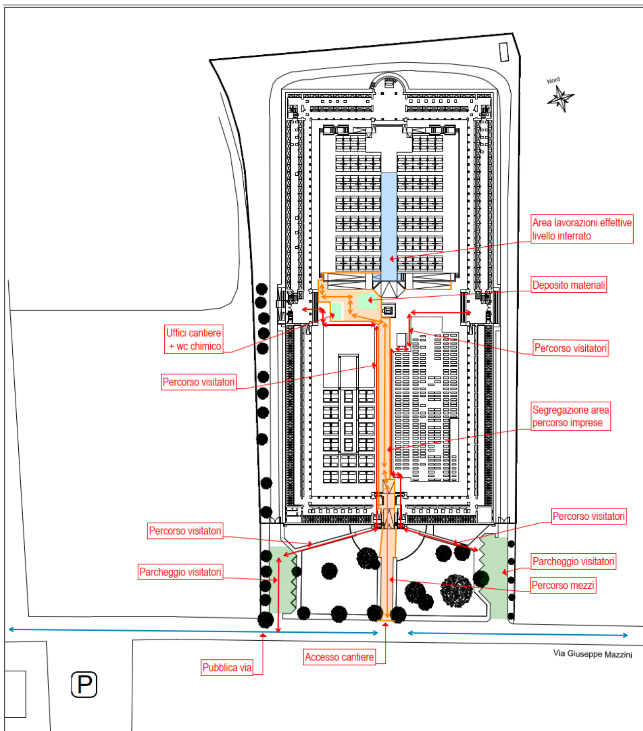
Indicazioni layout di cantiere
